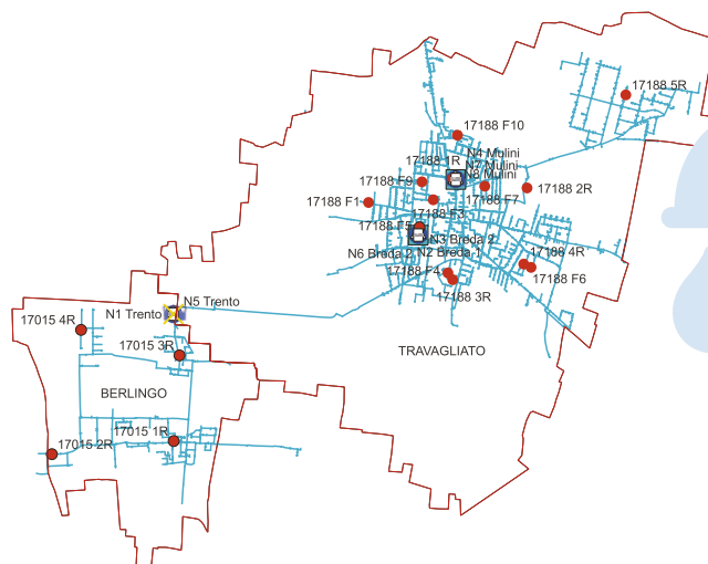
Sistema idropotabile georeferenziato di Berlingo-Travagliato Localizzazione nodi e internodi
